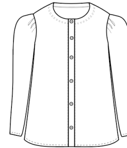
Puffärmel schmal
