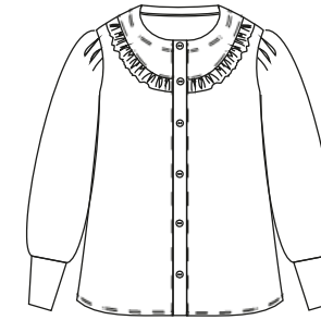
Bischofsärmel
