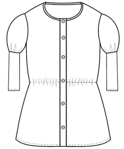
Ballonärmel
